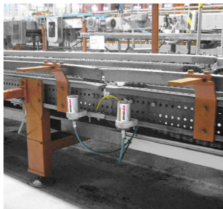
Två simalube med slangförlängning smörjer en transportörkedja i ett bryggeri.
